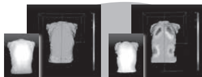
左右対称のデータ 左右非対称のデータ
